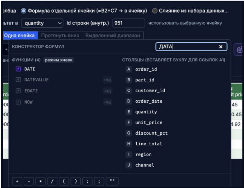
Поиск ДАТА показывает функцию DATE, доступную для формулы ячейки.
